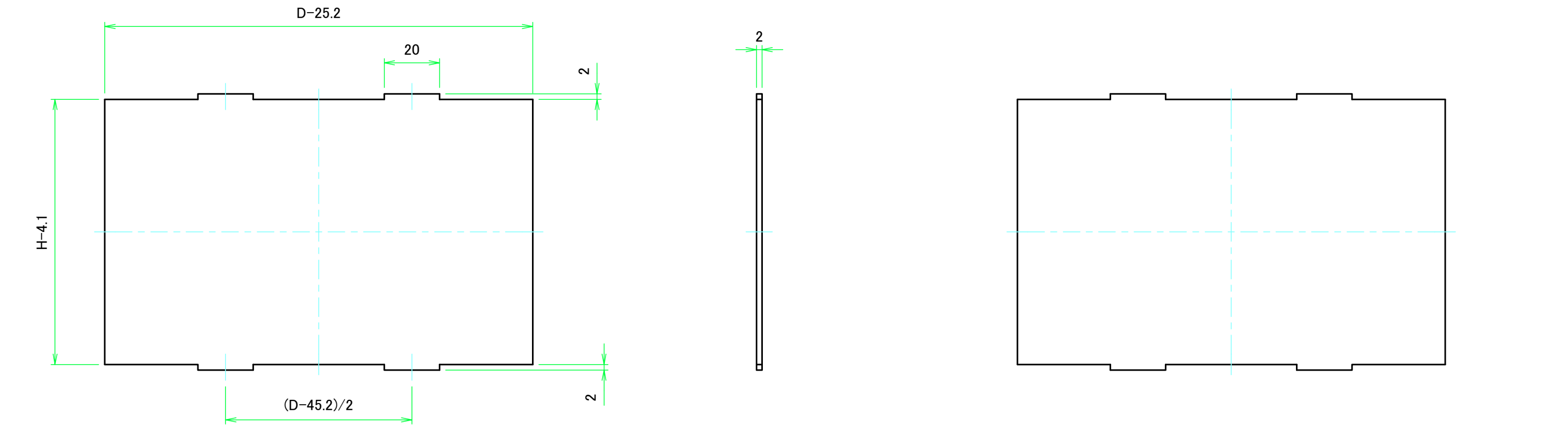
Dパネル1表面 / D Panel 1 Frontside
