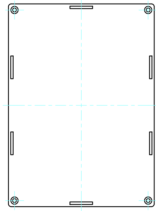
下カバー表面 / Bottom cover Frontside
